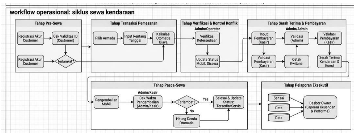
Gambar 2.3 Diagram Alur Kerja Aplikasi Rental Mobil
